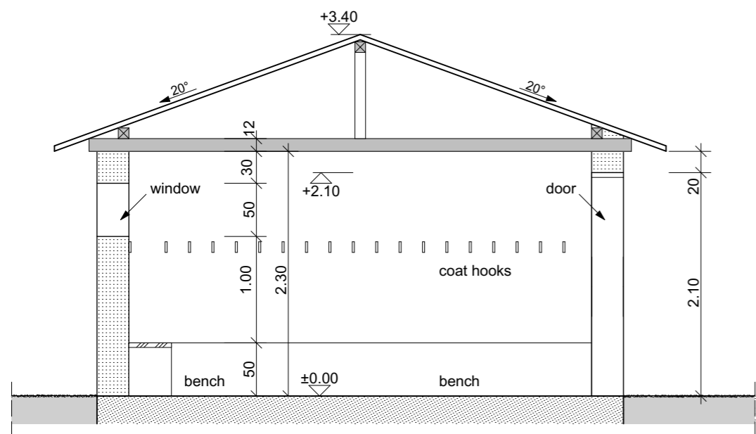
Schnitt 01
